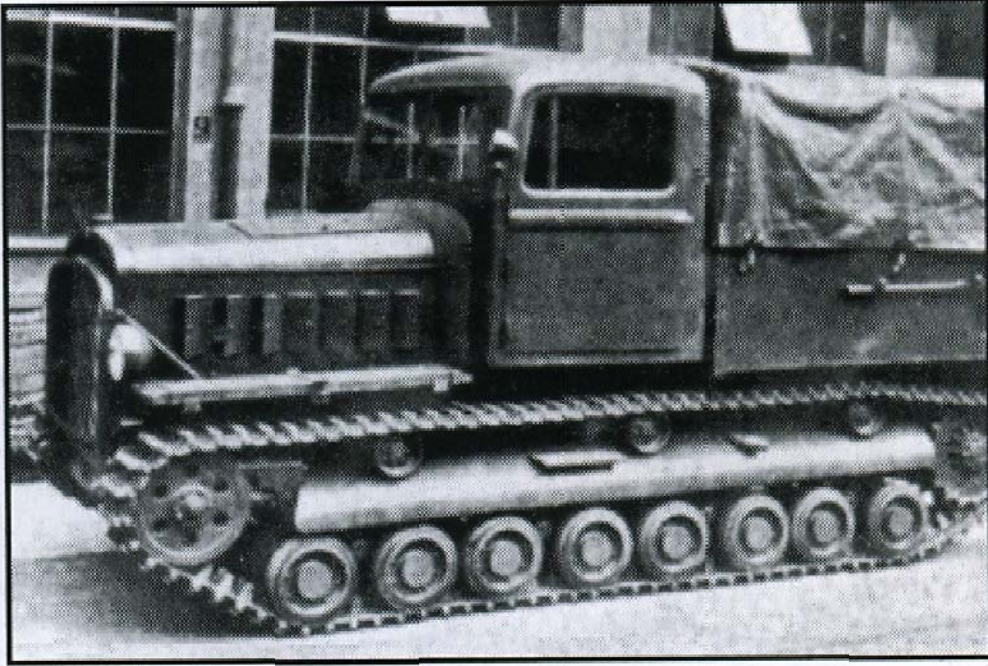
Traktor pásový Praga TH-T6
